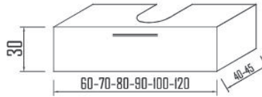
BAJO PORTALAVABO Con cajón extracción total
