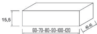
BASTIDOR SIN TAPA PARA ENCIMERA CERAMICA
